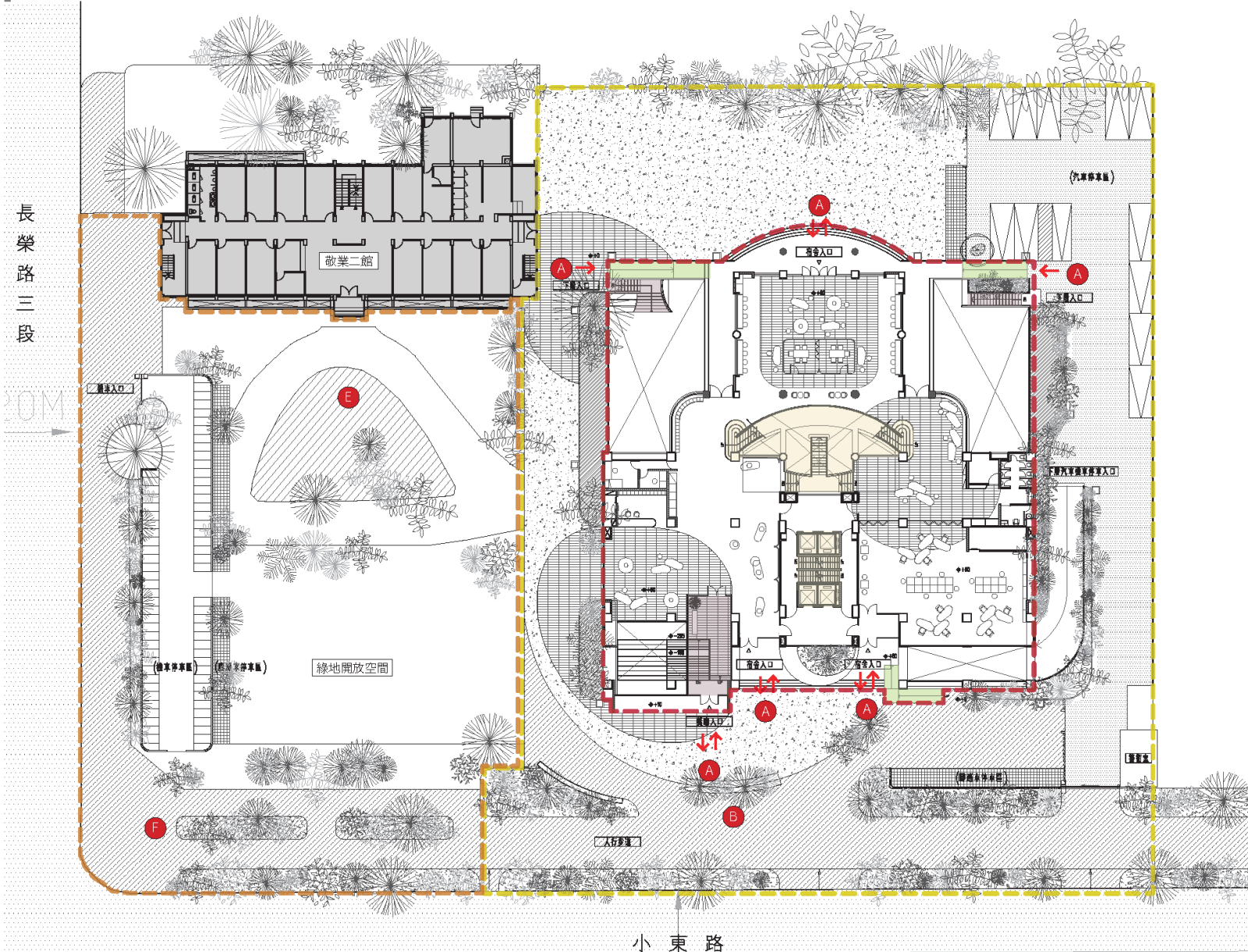
地面層平面圖 S:1/400
